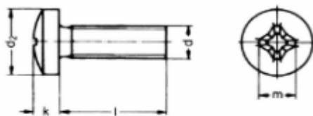
Linsenzylinder Schneidschraube Form A-h, Phillipskreuzschlitz H
